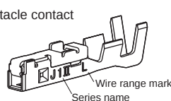
Receptacle contact
